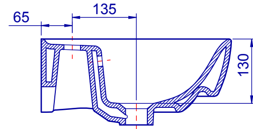
A-A KESİTİ
