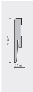
GP0601 60x15 mm SKIRTING 5905167766668 🚚2,42 m 📦24,2 m 🏠1161,6 m
