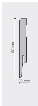
GP0801 80x15 mm SKIRTING 5905167766675 🚚2,42 m 📦24,2 m 🏠1016,4 m
