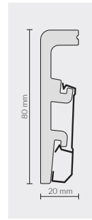
P0810 80x20 mm SKIRTING 5905167734551 2,4 m 24 m 504 m
