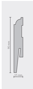
MP0901 90x15 mm SKIRTING 5905167674369 📏 2,42 m 📦 24,2 m 📦 847 m
