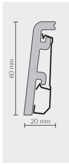
P0610 60x20 mm SKIRTING 5905167747926 2,4 m 24 m 672 m
