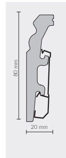
P0830 80x20 mm SKIRTING 5905167755679 2,4 m 24 m 504 m
