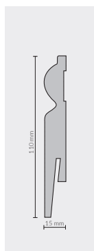
MP1101 110x15 mm SKIRTING 5905167674420 📏 2,42 m 📦 24,2 m 📦 847 m
