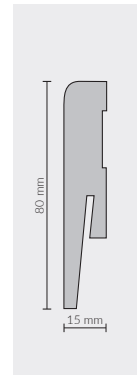
MP0801 80x15 mm SKIRTING 5905167674345 📏 2,42 m 📦 24,2 m 📦 847 m
