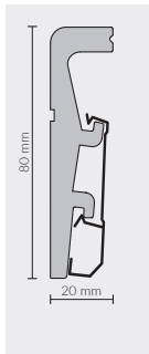
P0811 80x20 mm SKIRTING 5905167734568 2,4 m 24 m 504 m
